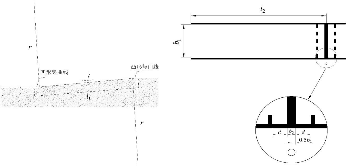
a) 截面图
