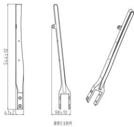
阶梯靠背左支撑件
