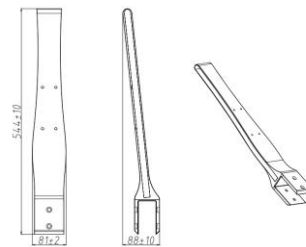
阶梯靠背中支撑件
