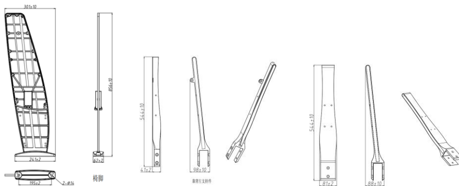
平面教室椅脚
